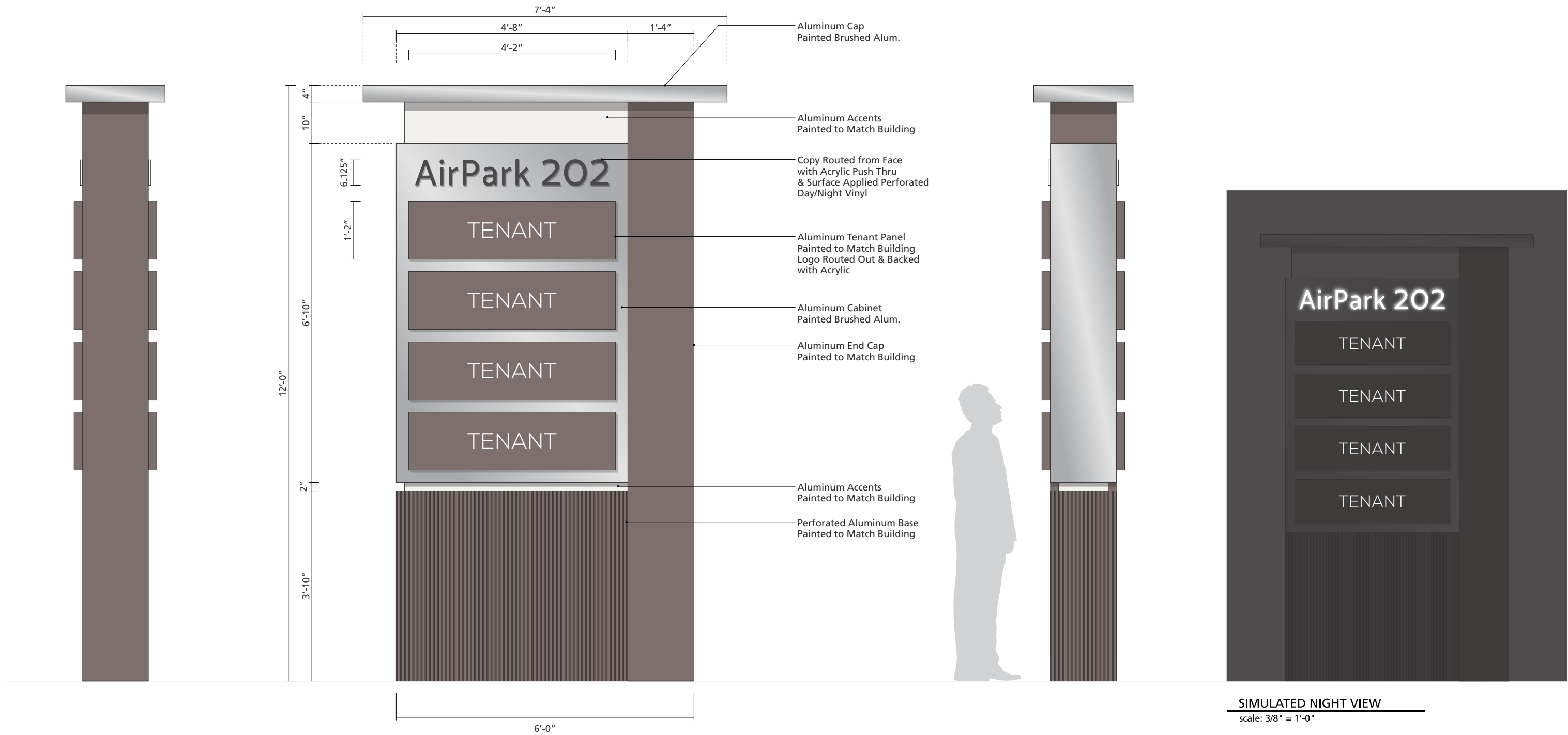
SIDE VIEW scale: 1/2" = 1'-0"
