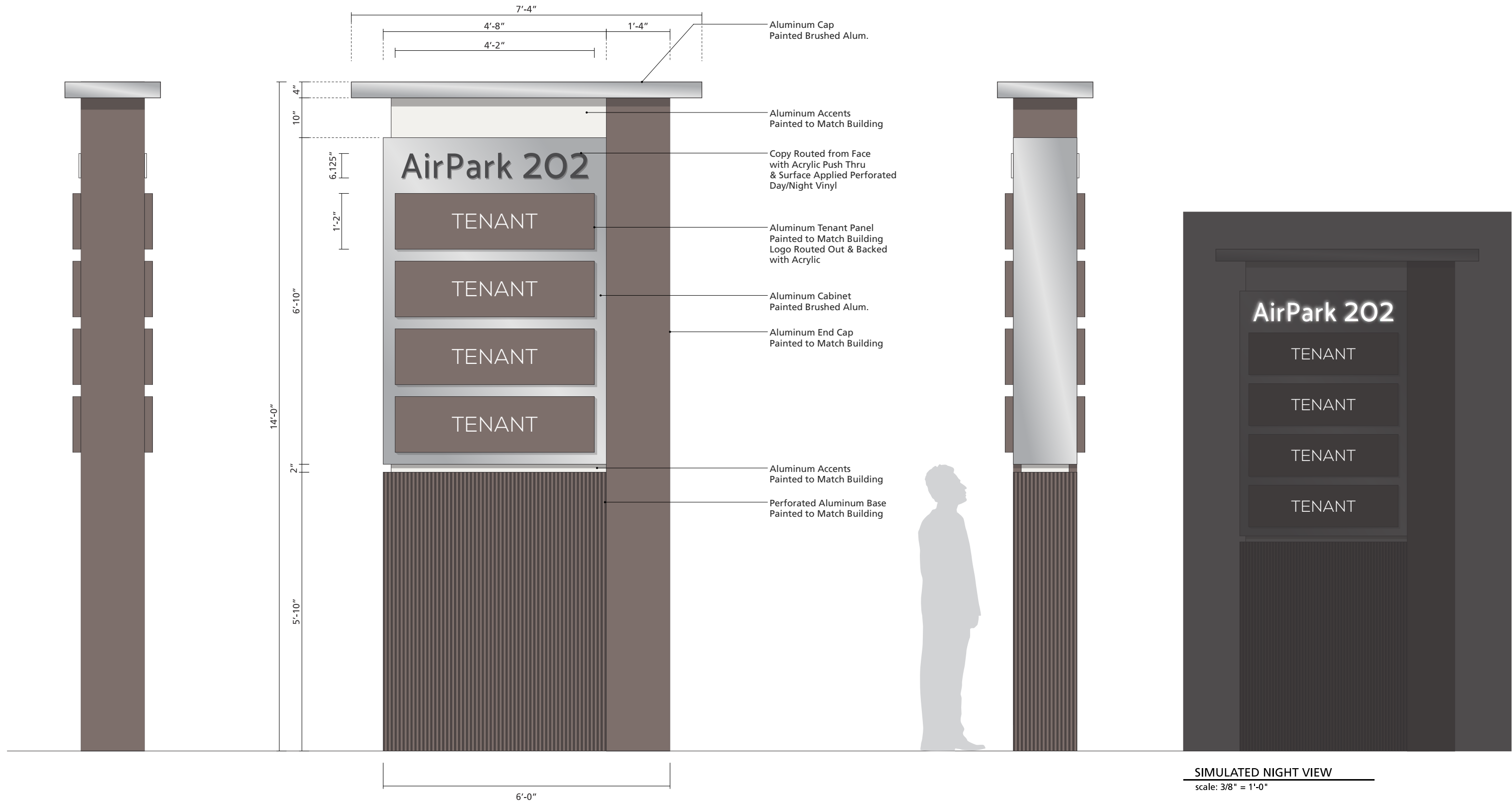
SIDE VIEW scale: 1/2" = 1'-0"
