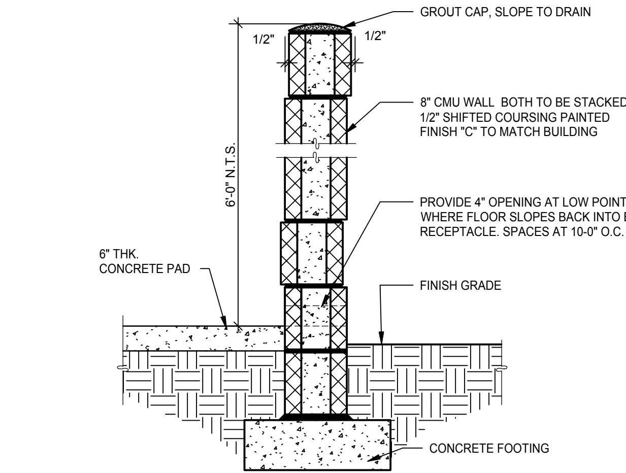
MASONRY TRASH WALL SCALE: 1" = 1'-0"
