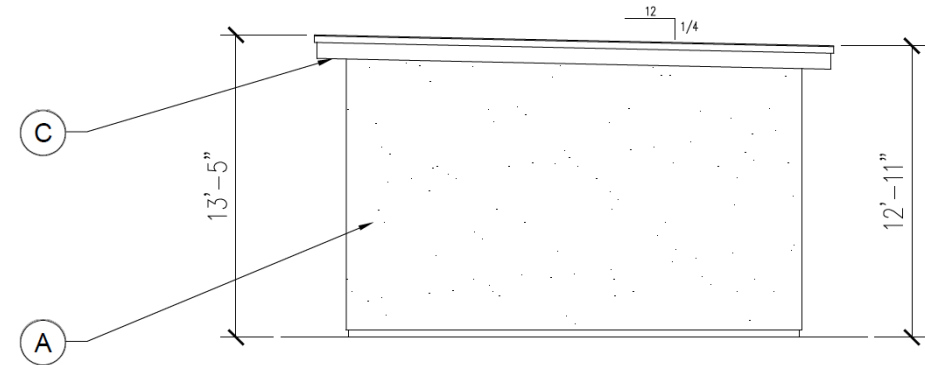
SIDE ELEVATION SCALE: 1/8" = 1'-0"
