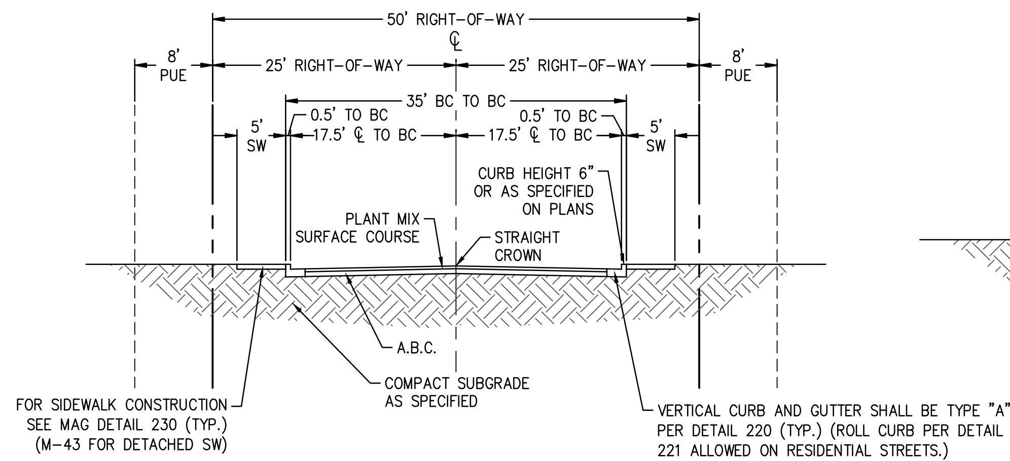
1 LOCAL STREET SECTION N.T.S.
