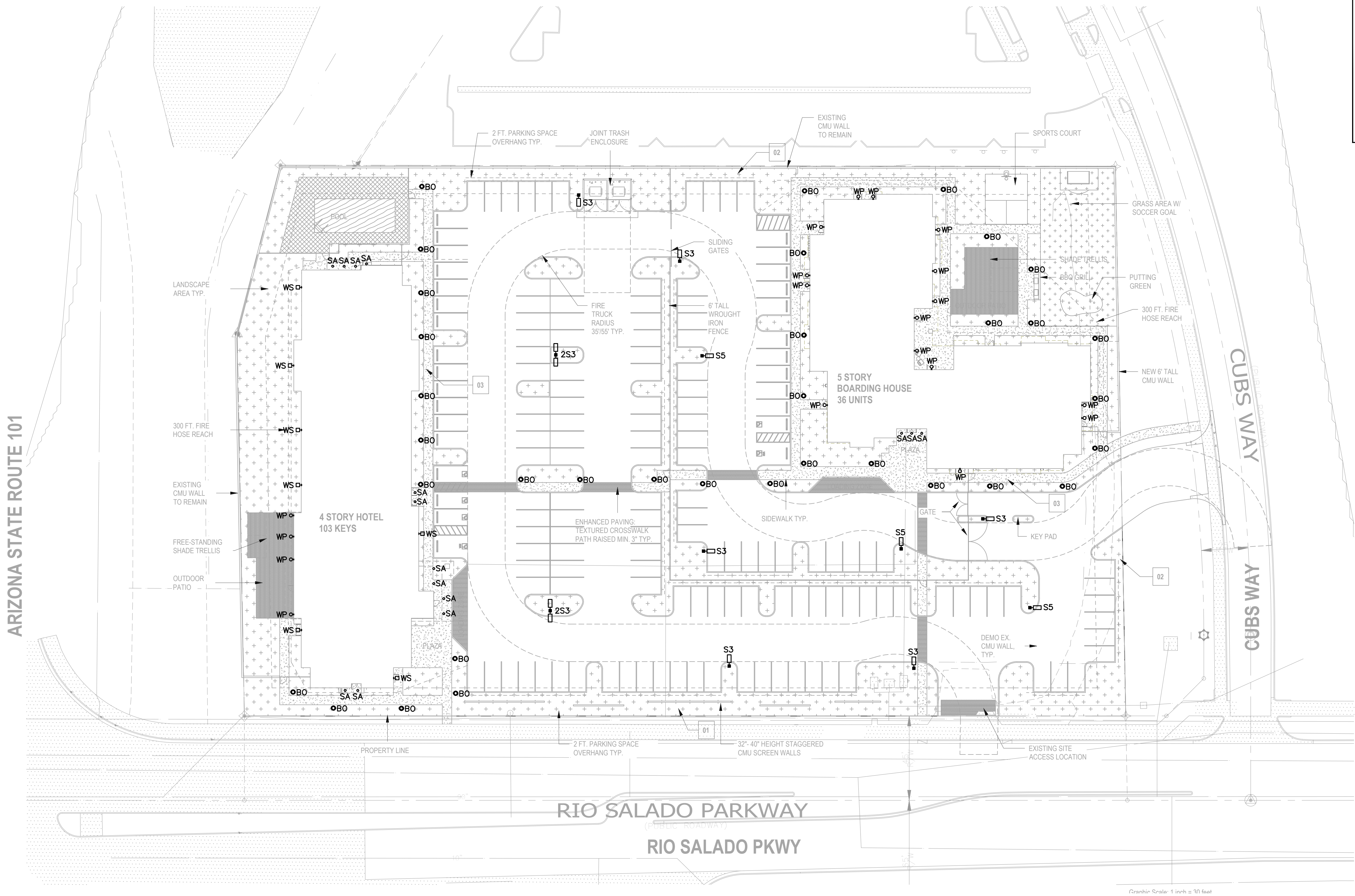
1 SITE LIGTING PLAN 1" = 30'-0"
