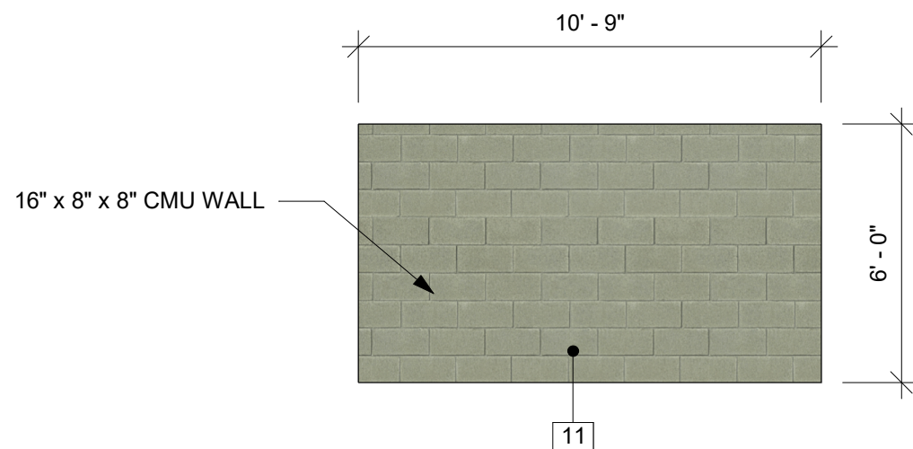
RIGHT ELEVATION
