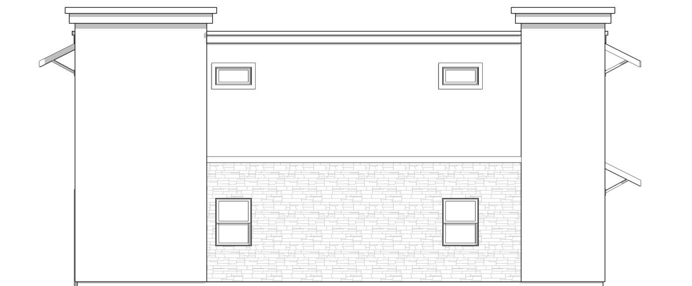
RIGHT ELEVATION
