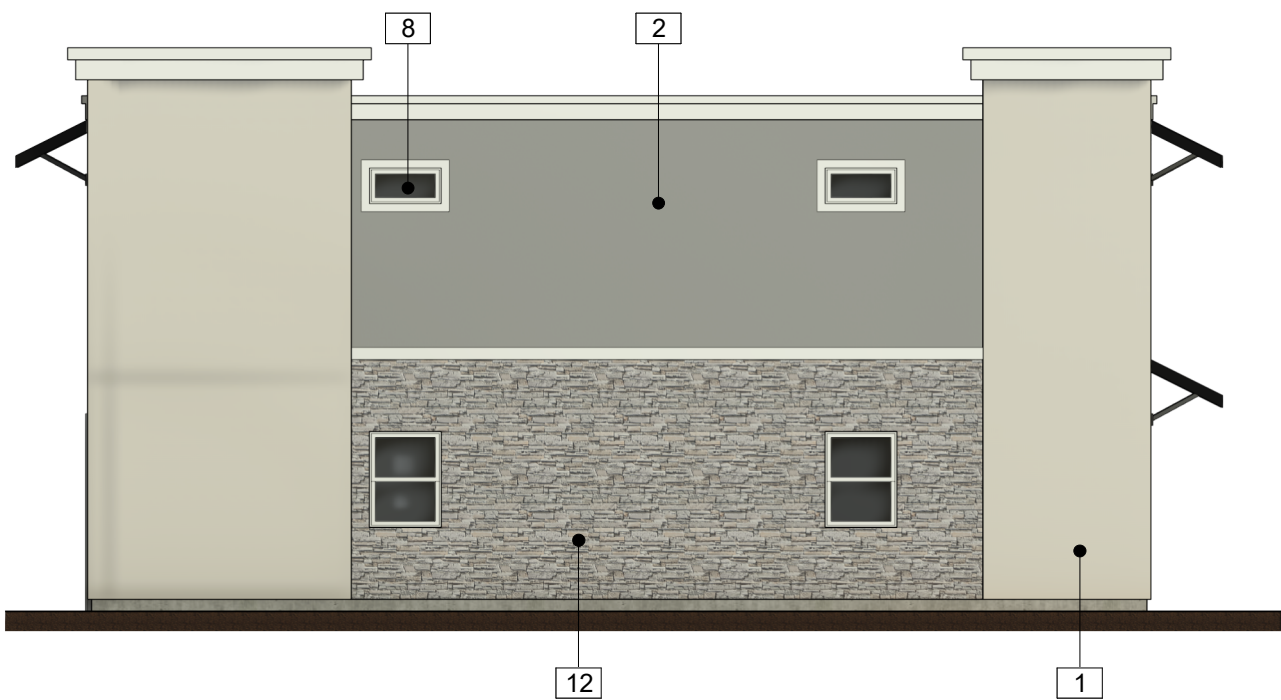
RIGHT ELEVATION
