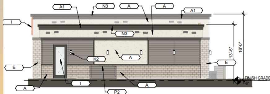
4 FITNESS - RIGHT ELEVATION A8 SCALE: 1/8" = 1'-0"
