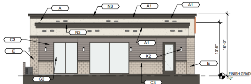
3 FITNESS - LEFT ELEVATION A8 SCALE: 1/8" = 1'-0"
