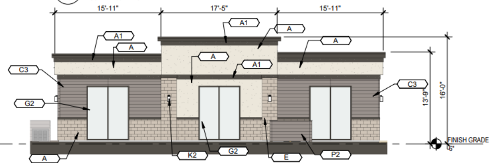
2 FITNESS CENTER - REAR ELEVATION A8 SCALE: 1/8" = 1'-0"
