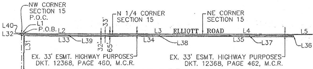
DETAIL "A" N.T.S.
