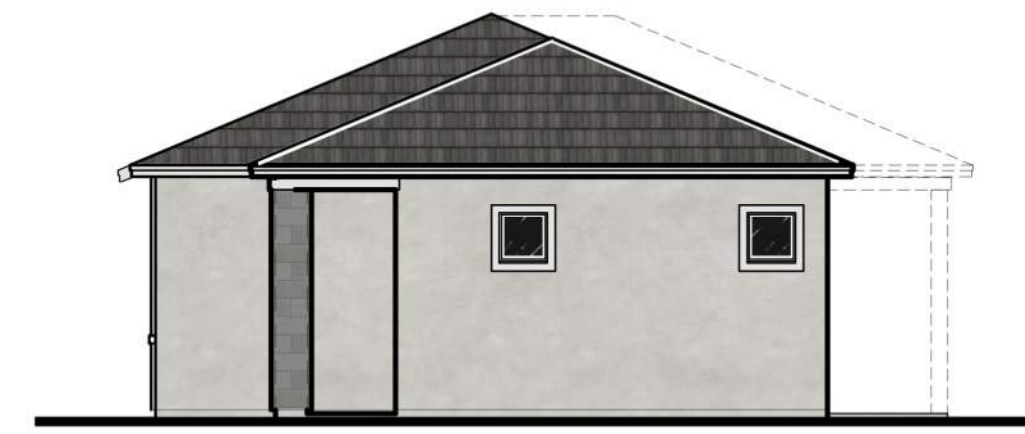
Right Elevation
